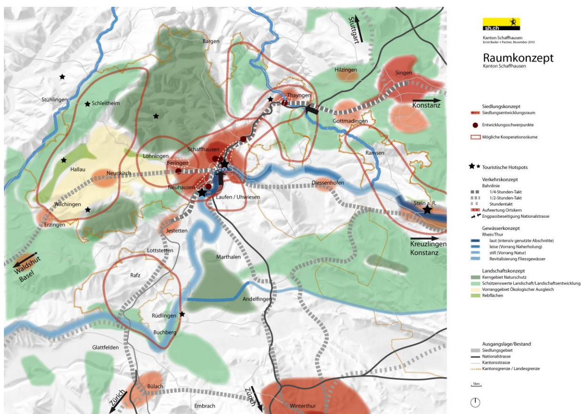
Abbildung 33: Gültiges Raumkonzept Kanton Schaffhausen, Quelle: Fachstelle Raumplanung Kanton Schaffhausen
