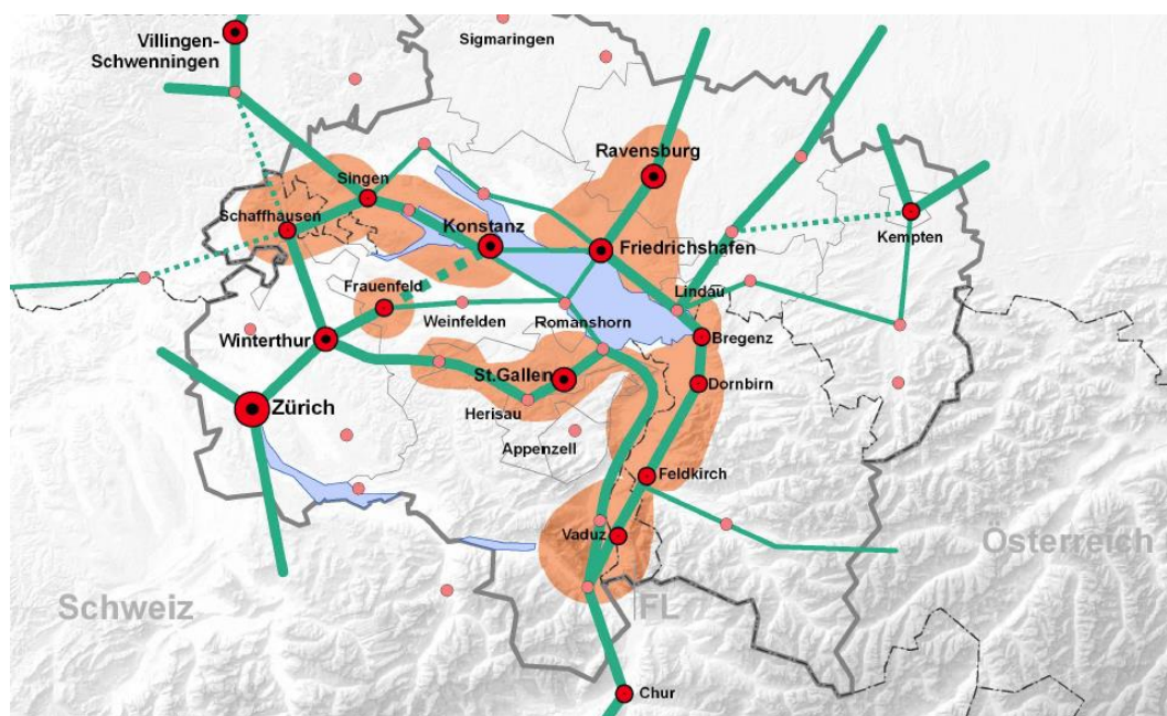
Abbildung 17: Funktionsräumliche Aufteilung Ostschweiz – heterogener Wirtschaftsraum, Quelle: Universität St. Gallen, 2014, Perspektiven für den Wirtschaftsraum Ostschweiz
