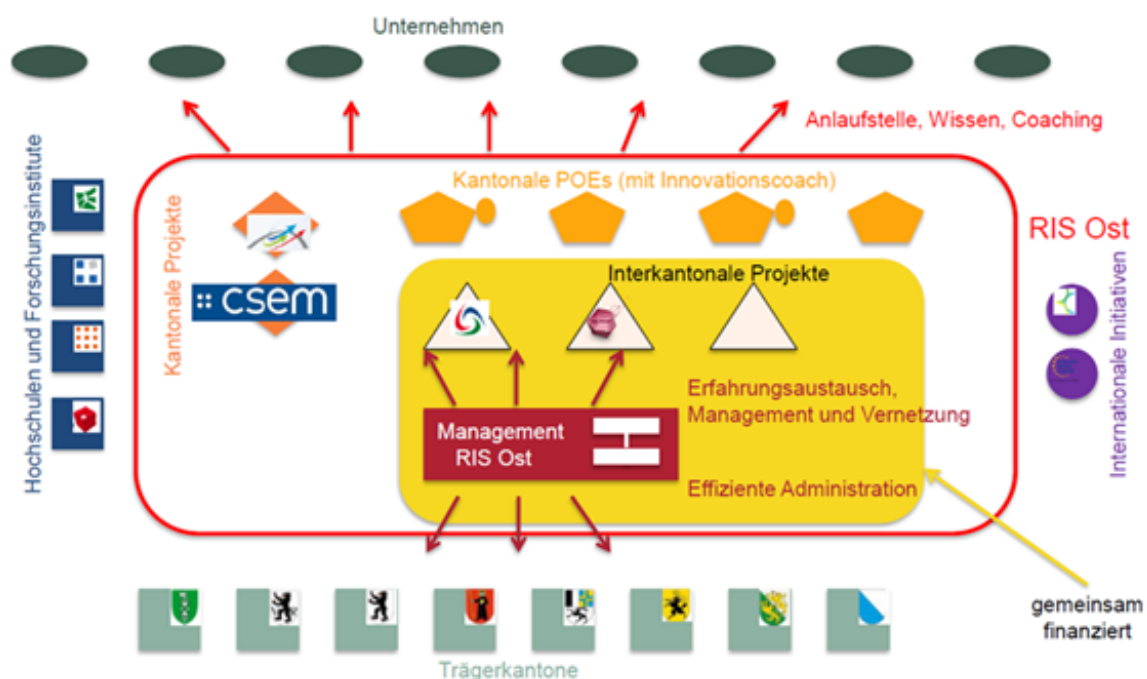
Abbildung 35: Regionales Innovationssystem Ostschweiz RIS Ost, Quelle: BHP Hanser und Partner, 2015
